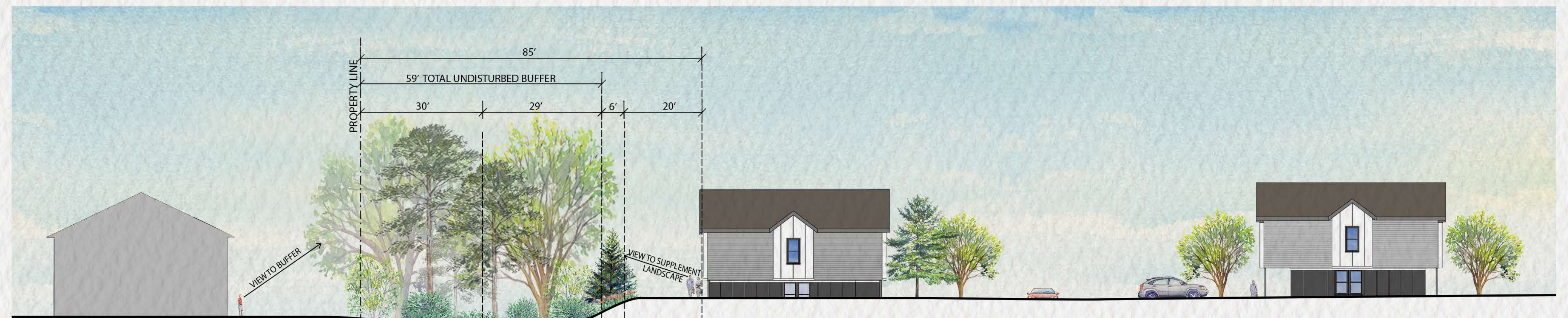
3 3-3 SECTION scale: 1"=16'-0"
